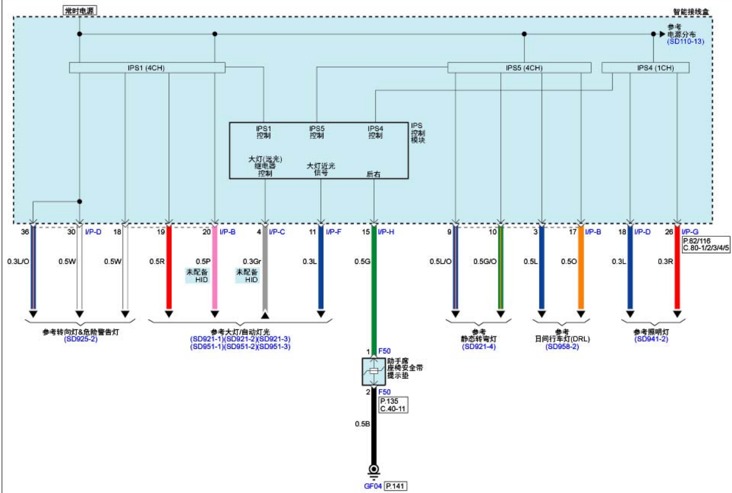
智能电源开关(IPS)系统(3)
